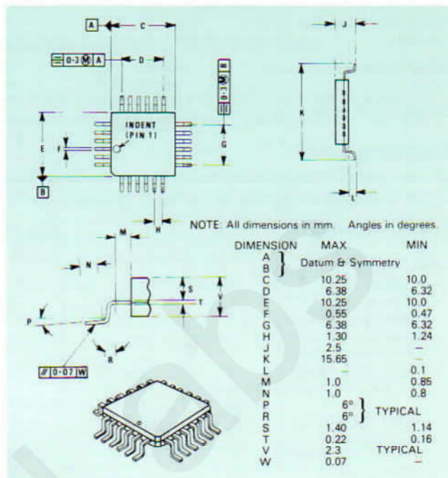
Fig. 7 FX004LG Package
