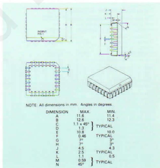
Fig. 8 FX004LH Package
