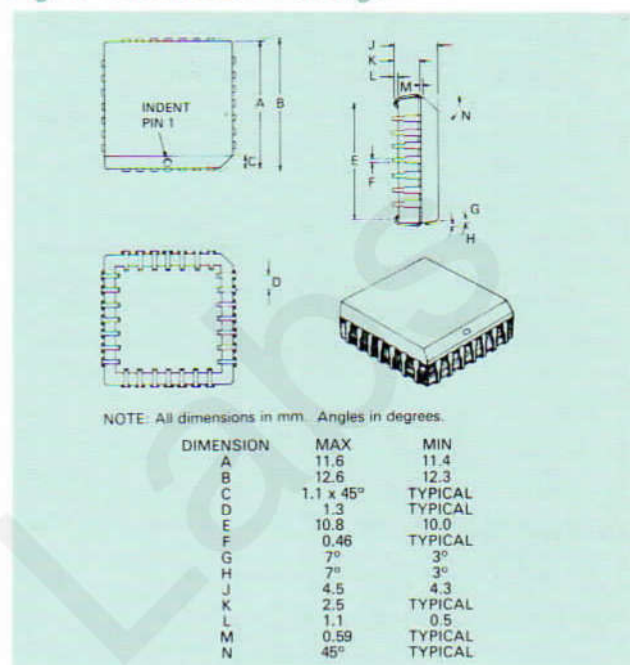
Fig. 9 FX204LH Package
